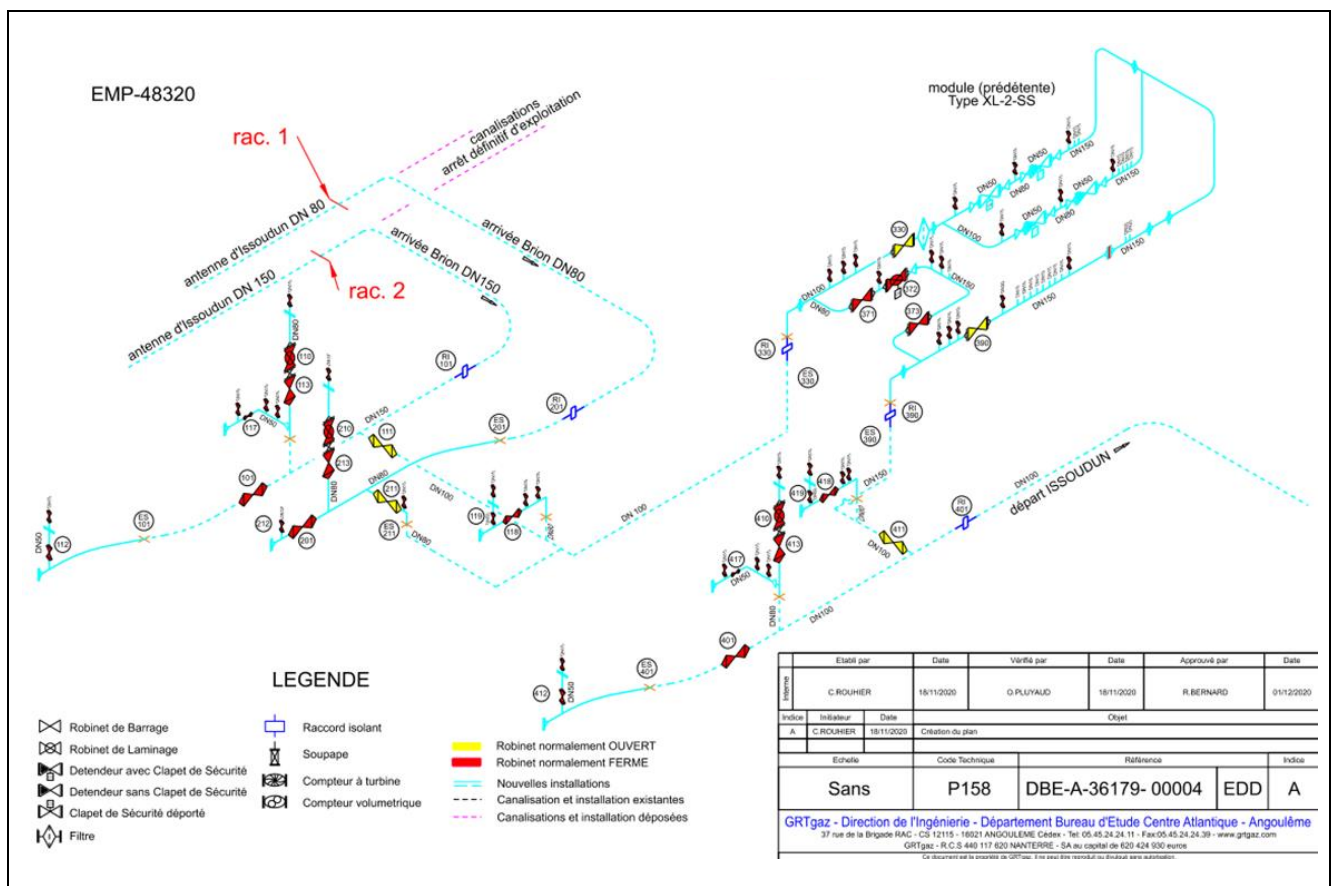
Figure 5 : Vue isométrique de l'installation annexe - Poste de Saint-Aoustrille
