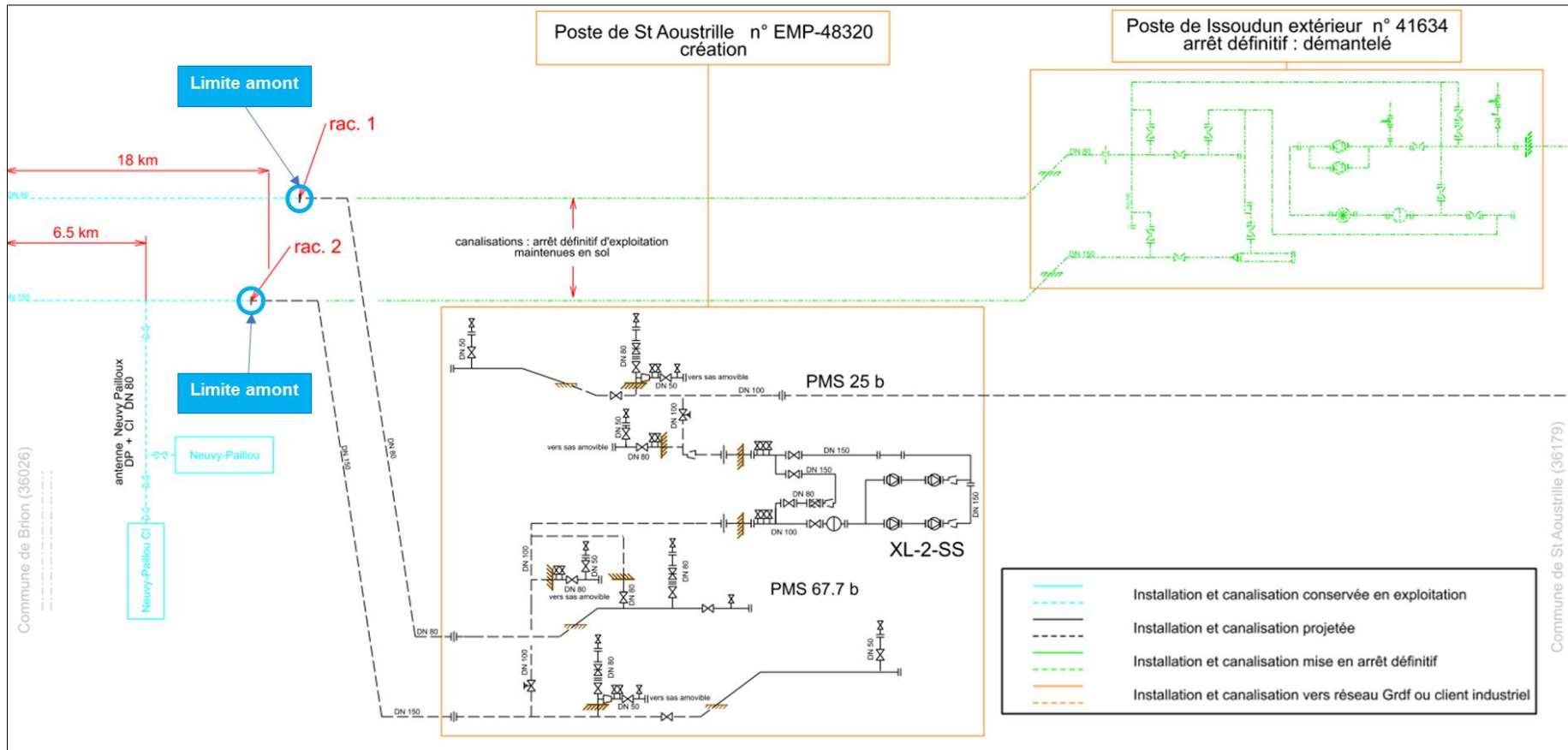
Figure 3 : Schéma d'armement de l'ouvrage projeté (1/2)
