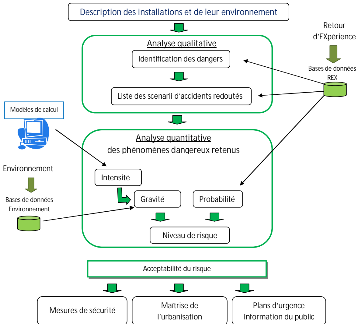
Figure n° 16 : Logigramme de la méthodologie d'analyse des risques
