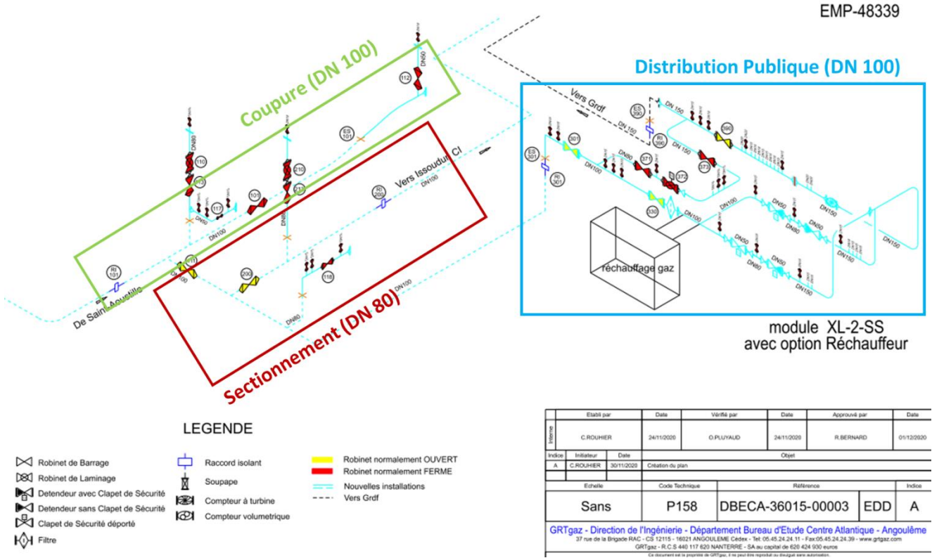
Figure 9 : Découpage en installations annexes simples du poste d'Issoudun
