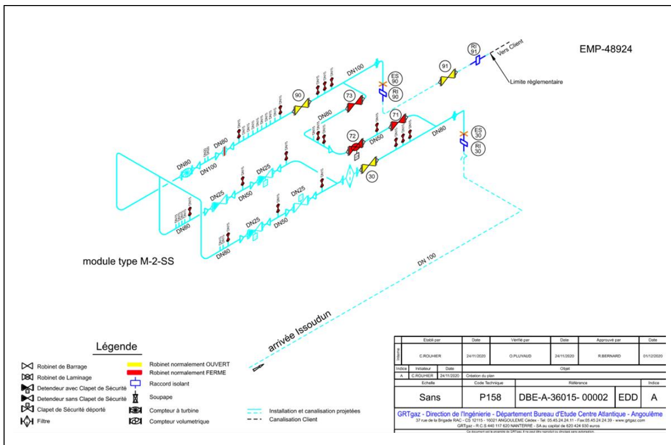
Figure 7 : Vue isométrique de l'installation annexe - Poste d'Issoudun CI Chaufferie
