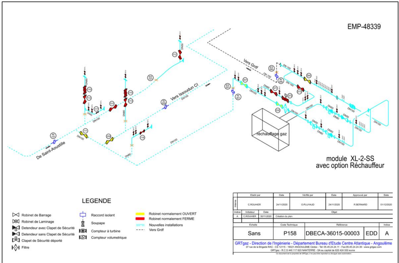
Figure 6 : Vue isométrique de l'installation annexe - Poste d'Issoudun (distribution publique)
