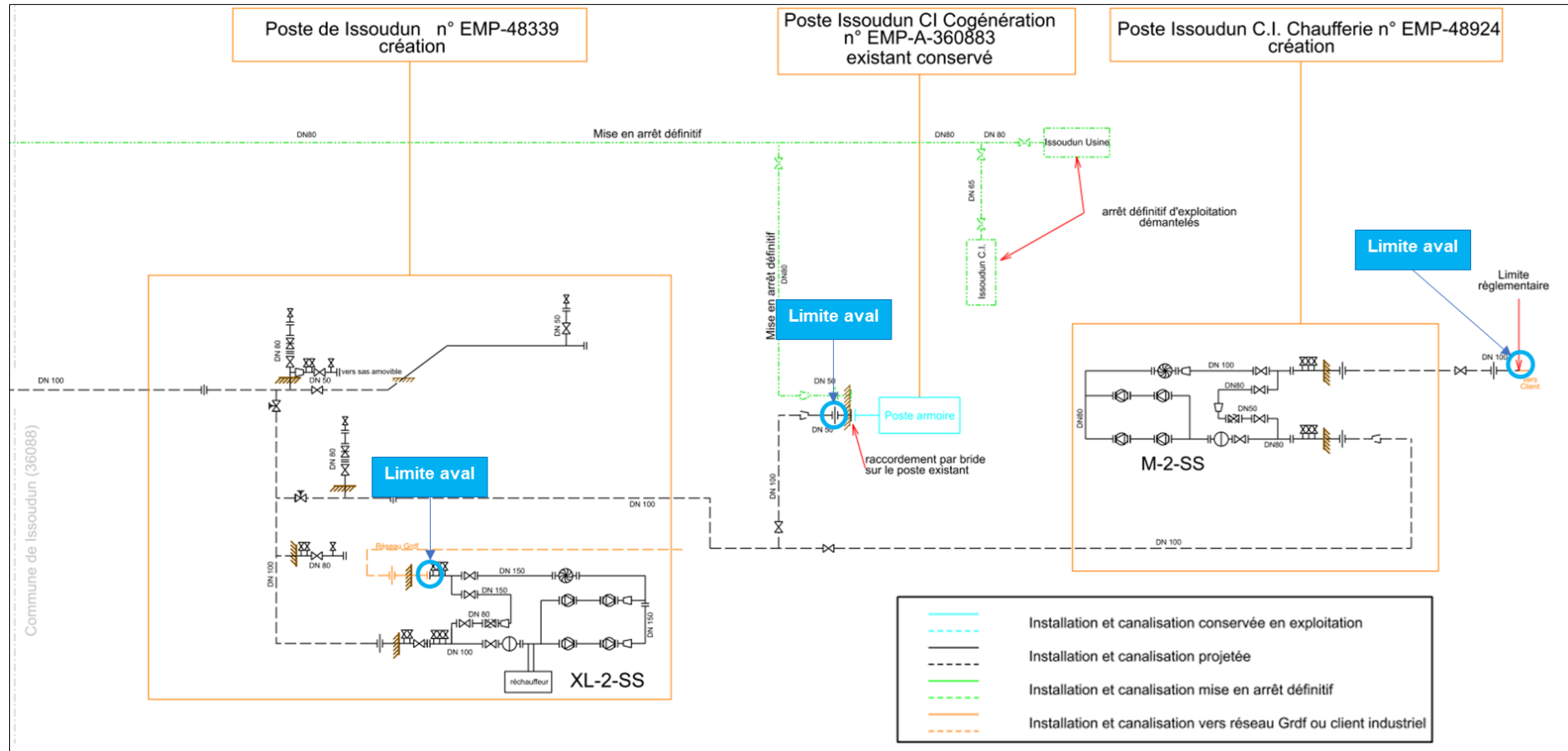
Figure 4 : Schéma d'armement de l'ouvrage projeté (2/2)
