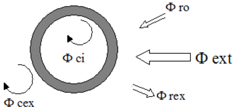
Figure 6 : Flux de chaleur sur une canalisation soumise à un rayonnement
