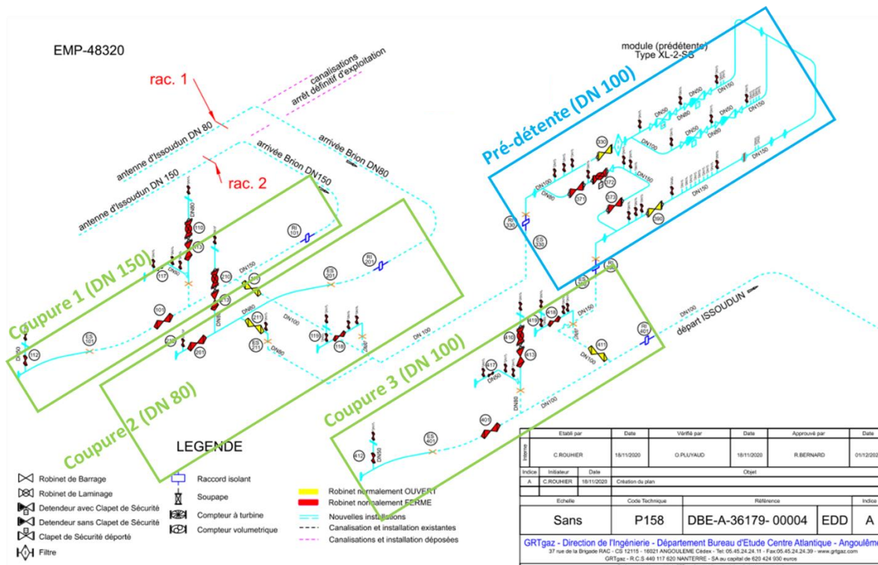
Figure 8 : Découpage en installations annexes simples du poste de Saint-Aoustrille
